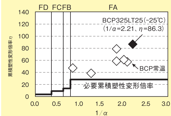
等価幅厚比 - 累積塑性変形倍率の関係
