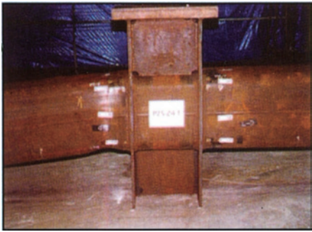
試験終了後：600×600×25 (mm) 試験体
