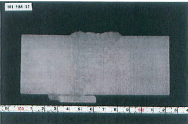
柱ー柱溶接 マクロ写真（平板部）
