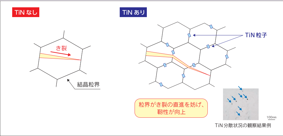
TiNの効果の模式図
