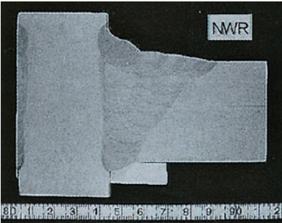
柱ー通しダイアフラム溶接部
