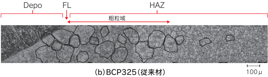
CO 2 溶接 熱影響 (HAZ) 部の組織比較
