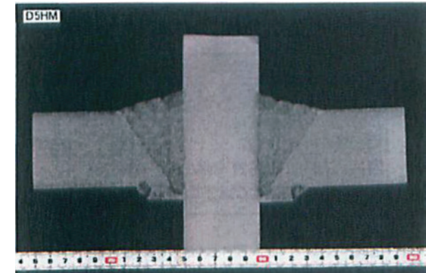
柱ー通しダイアフラム溶接 マクロ写真（平板部）
