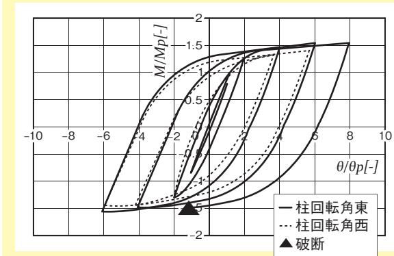
基準化曲げモーメントと回転角の関係
